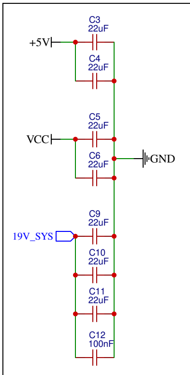
Decoupling Caps
